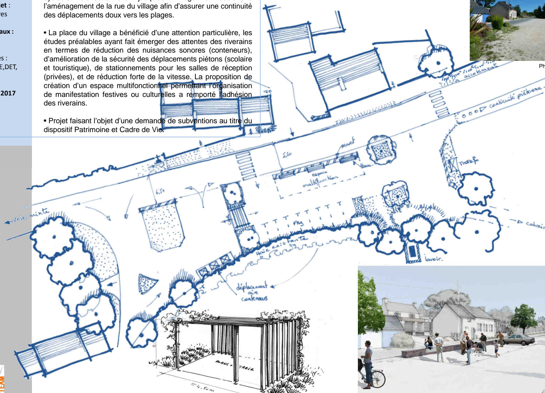
Croquis de l'abris mutualisé, entre l'arrêt de car et la place, évitant de cloisonner l'espace
